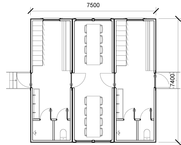
Plan 1 1 : 100
