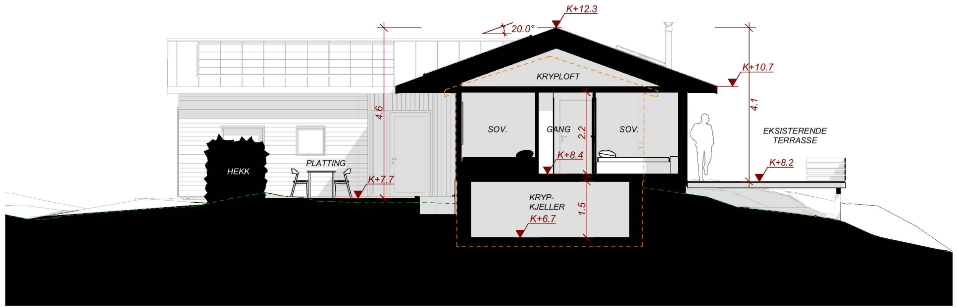
Snitt B - Planlagt
