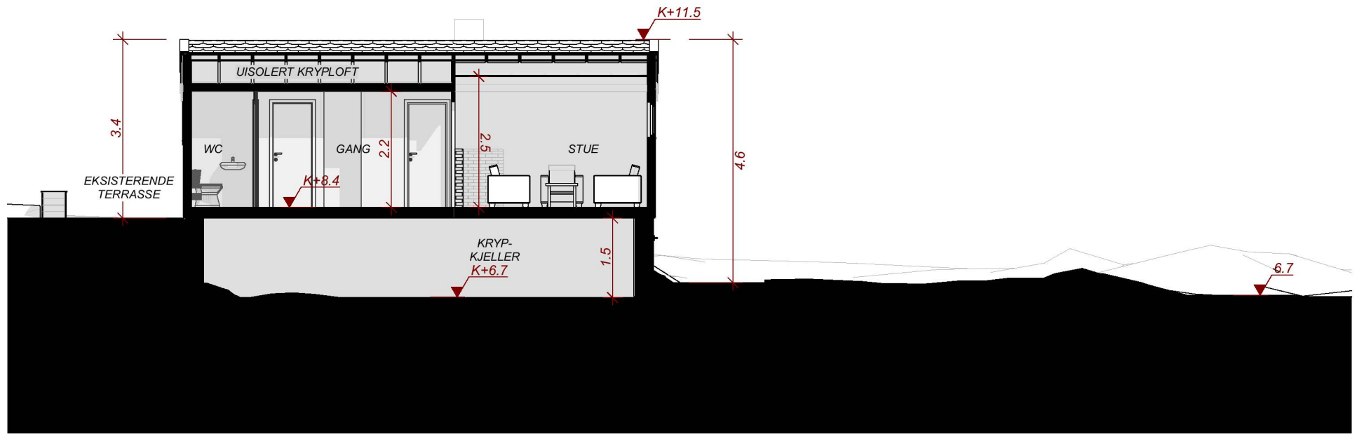
Snitt D - Eksisterende
