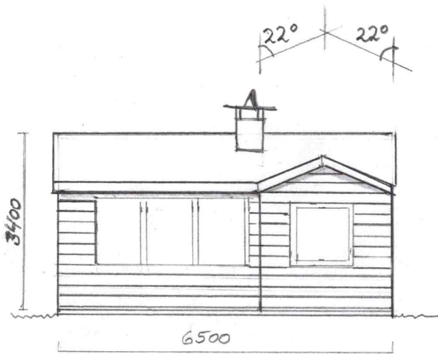
FASADE S
