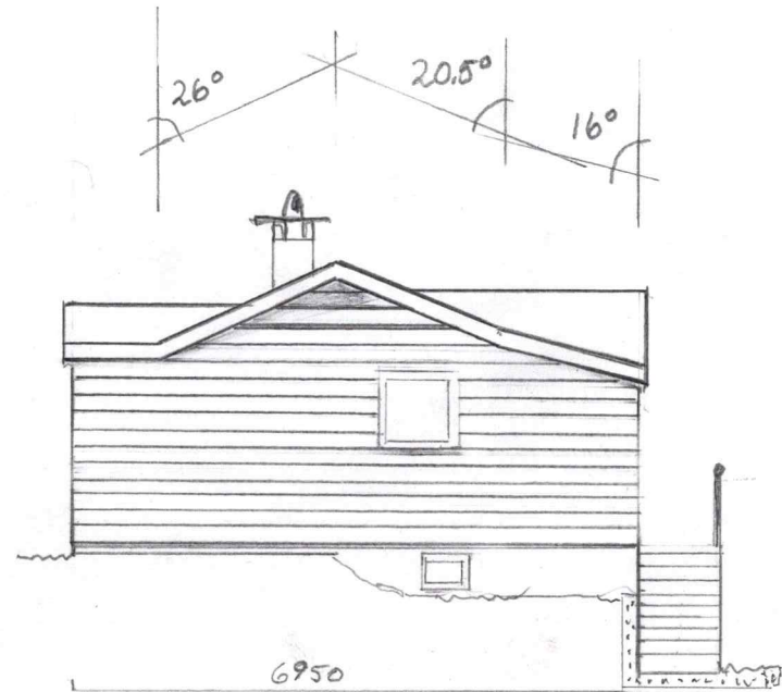
FASADE Ø
