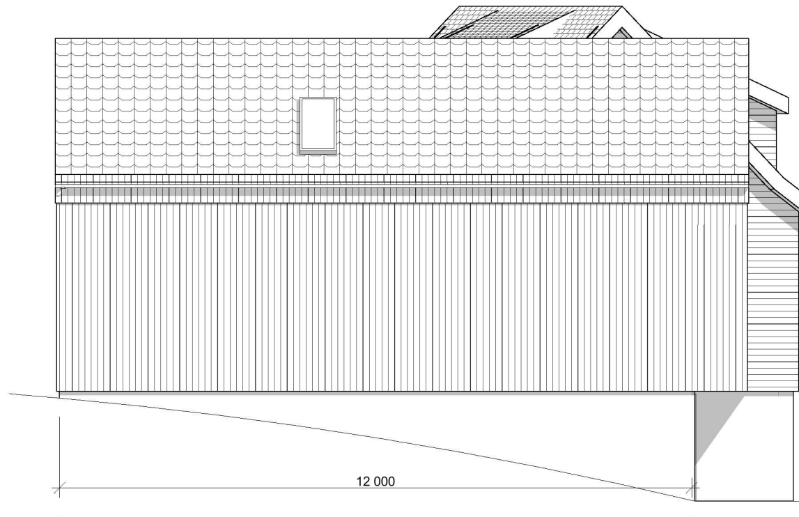
1:100 Fasade Vest
