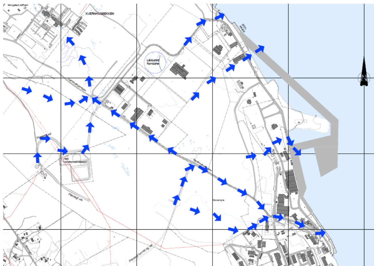
Figur 14: Planlagde flomvegar. Utsnitt av VA masterplan (ref. rapport frå Norconsult)
