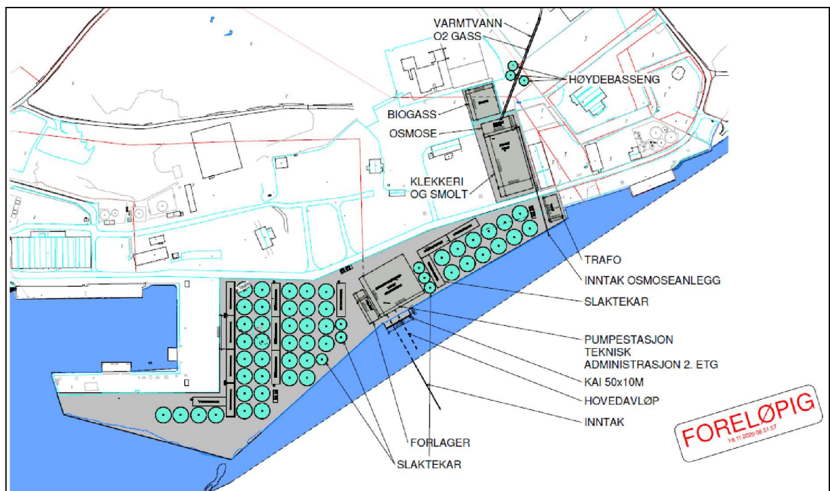
Figur 7: Mongstad Base 2D. Kjelde: Multiconsult AS. Planen er ein foreløpig illustrasjon.
