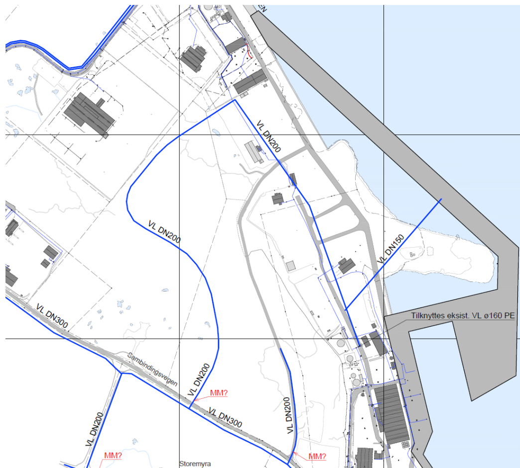
Figur 8: Planlagde vassleidninger. Utsnitt av VA masterplan (ref. rapport frå Norconsult)
