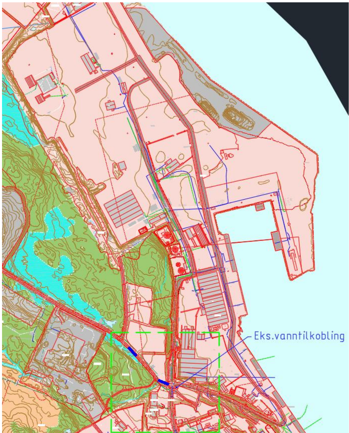
Figur 3: Utsnitt av Alver kommune sitt VA kart
