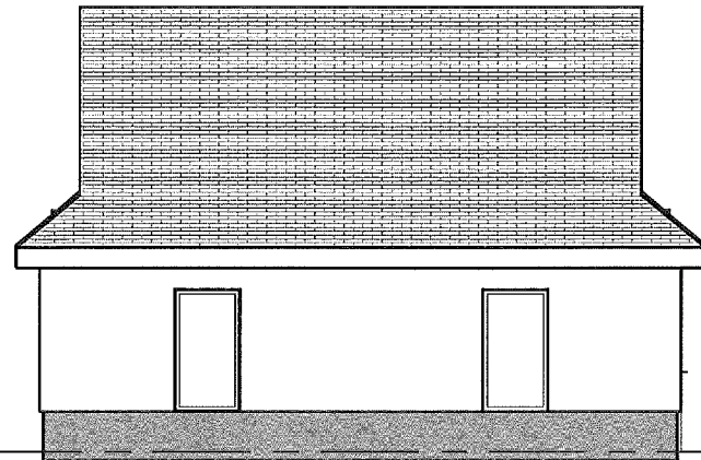
1 Fasade nordvest 1 : 100
