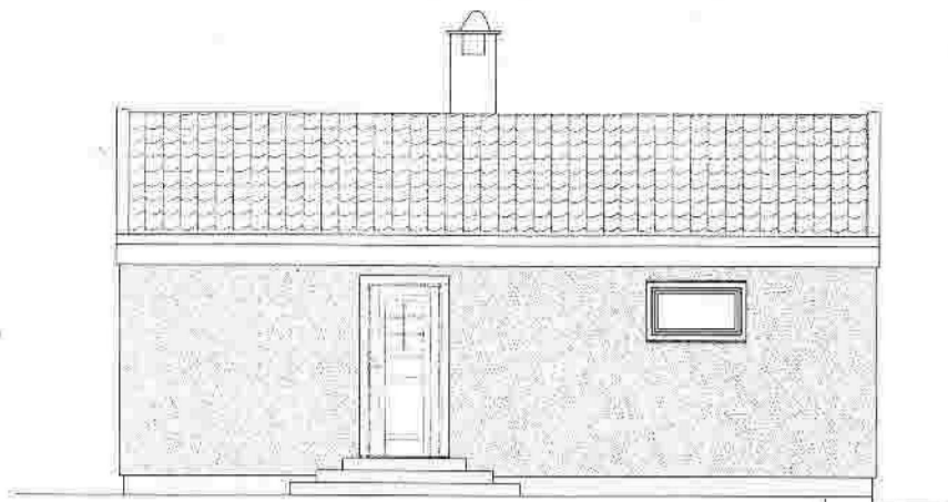
FASADE MOT NORDØST FØR ENDRING
