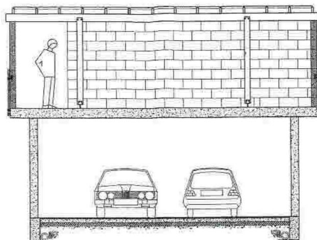
SNITT B-B MÅL 1:100
