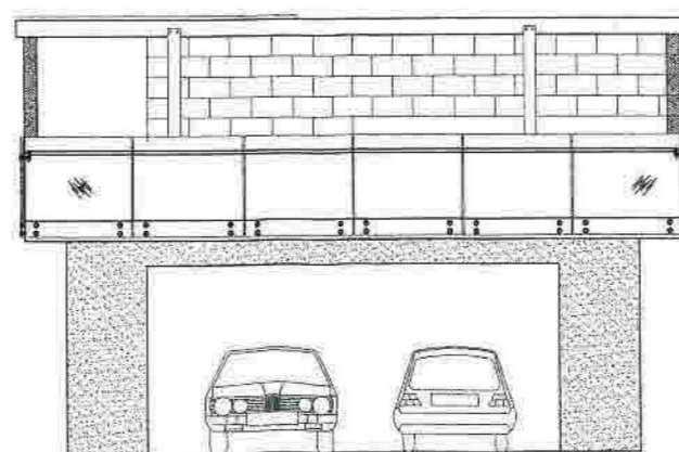
FASADE MOT SØRVEST MÅL 1:100
