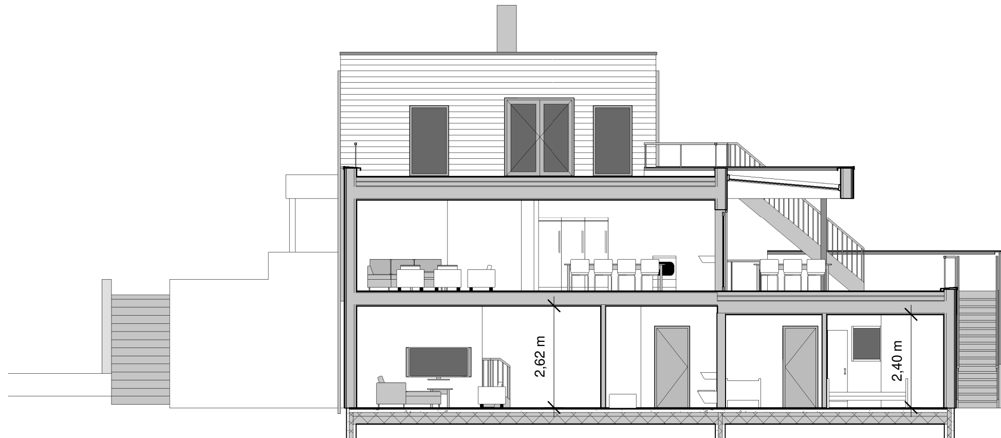
1 Langsnitt tilbygg 1 : 100
