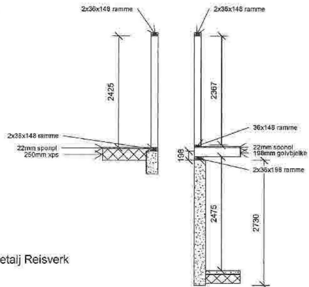
Snitt A
