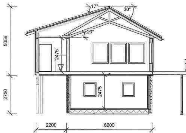
Snitt A
