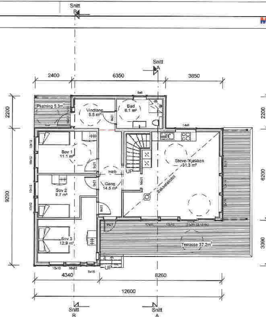
01 plan 1 Etasje
