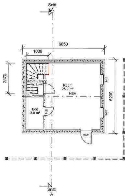
00 Plan Kjeller
