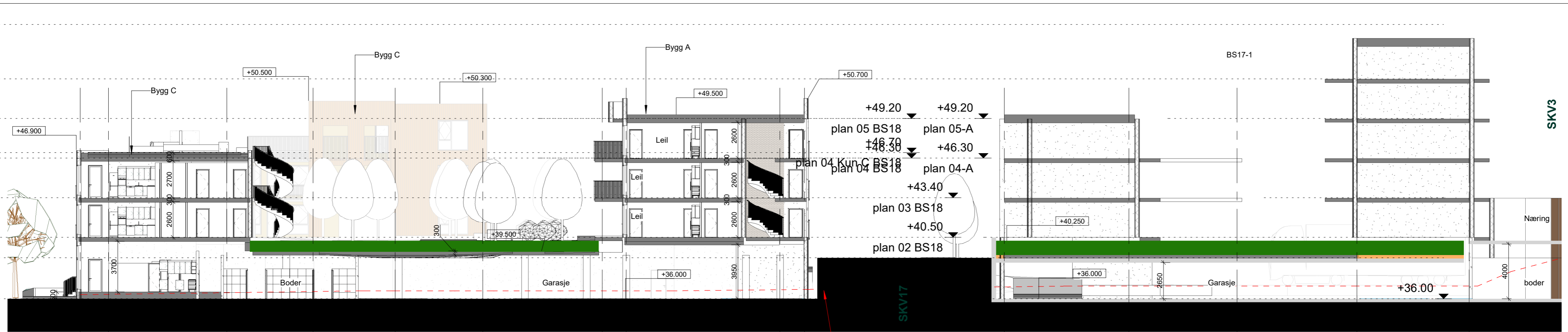
Snitt A
