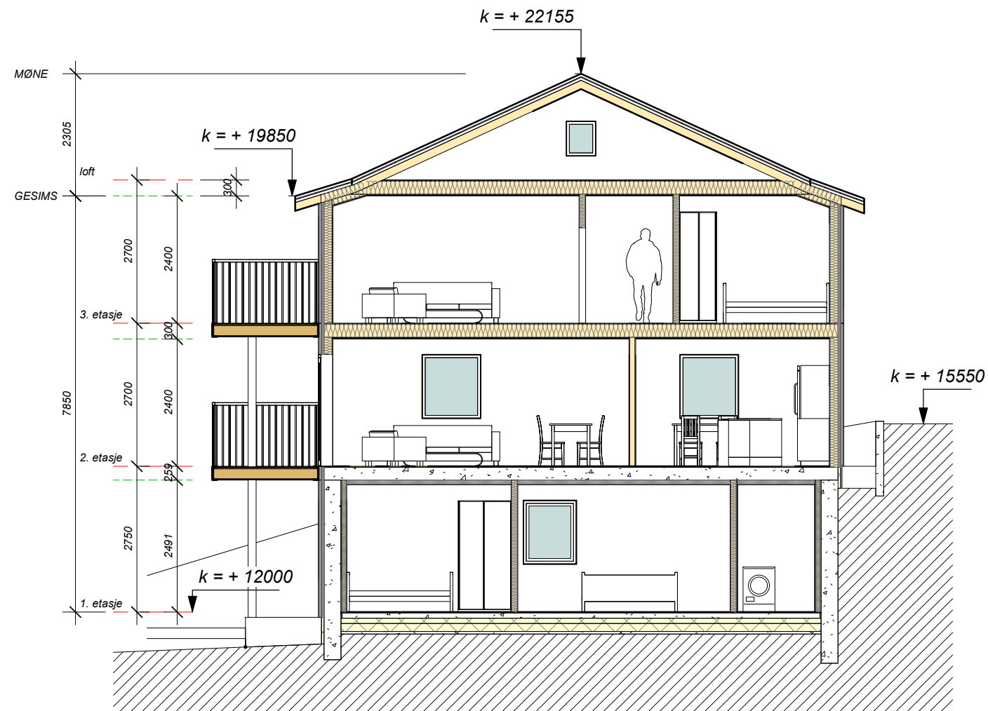
1 Snitt A-A 1 : 100
