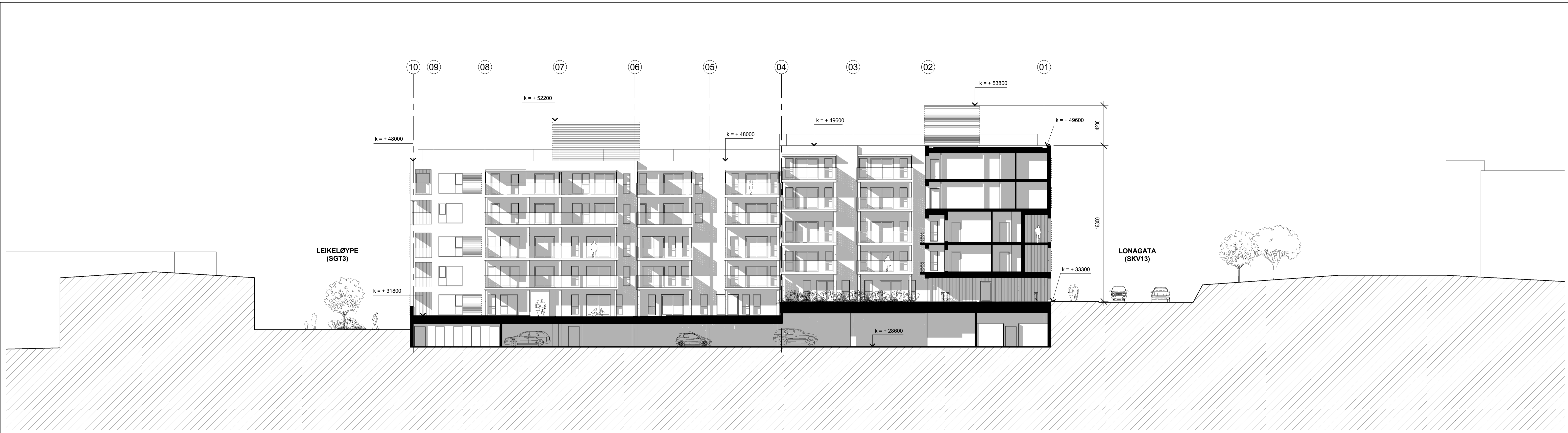
1 Terrengsnitt 1-1 1 : 200
