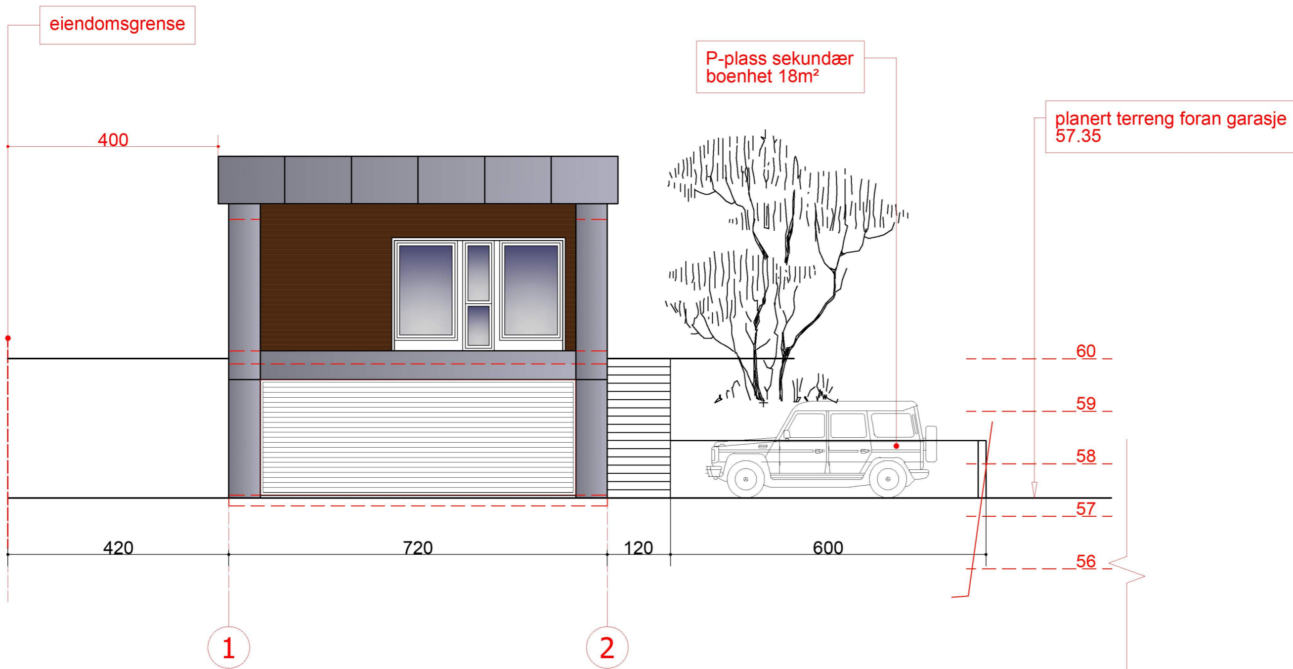
FASADE NORD
