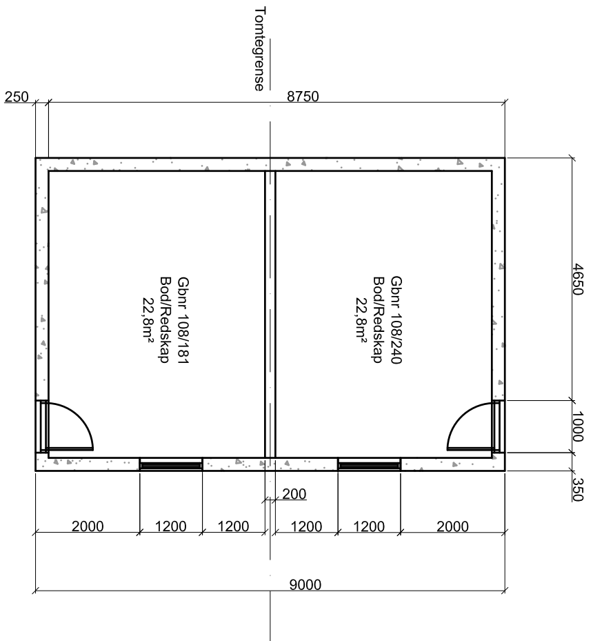
Plan 1. etasje
