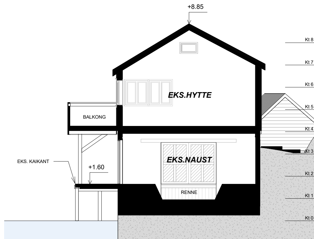
EKS. SNITT B-B' 1:100
