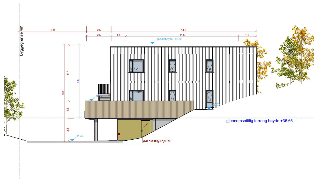
Hus C Fasade Nord 1:200
