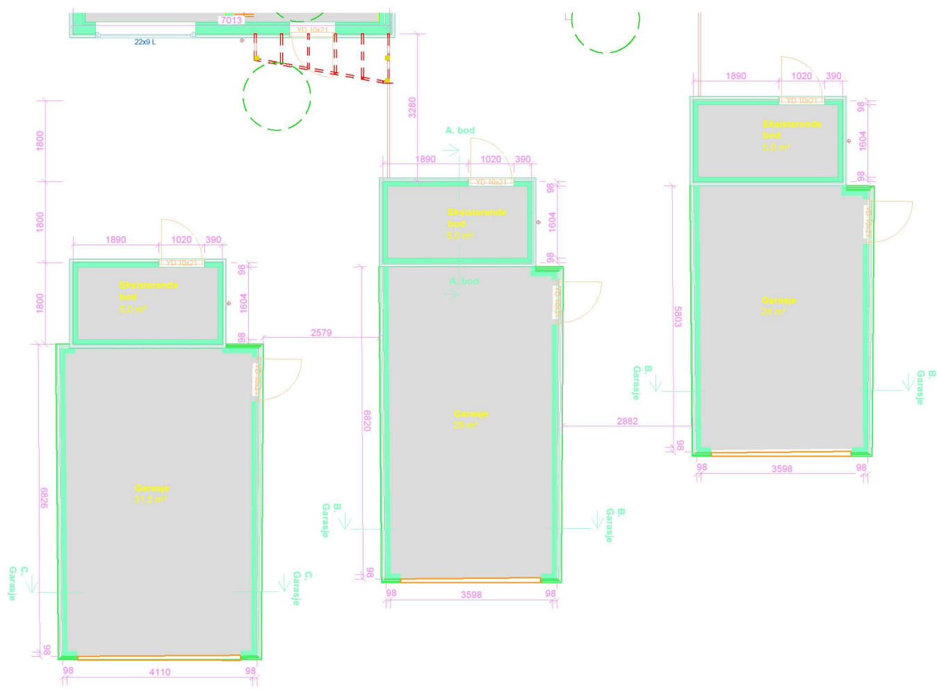
Plantegning Målestokk 1 : 100
