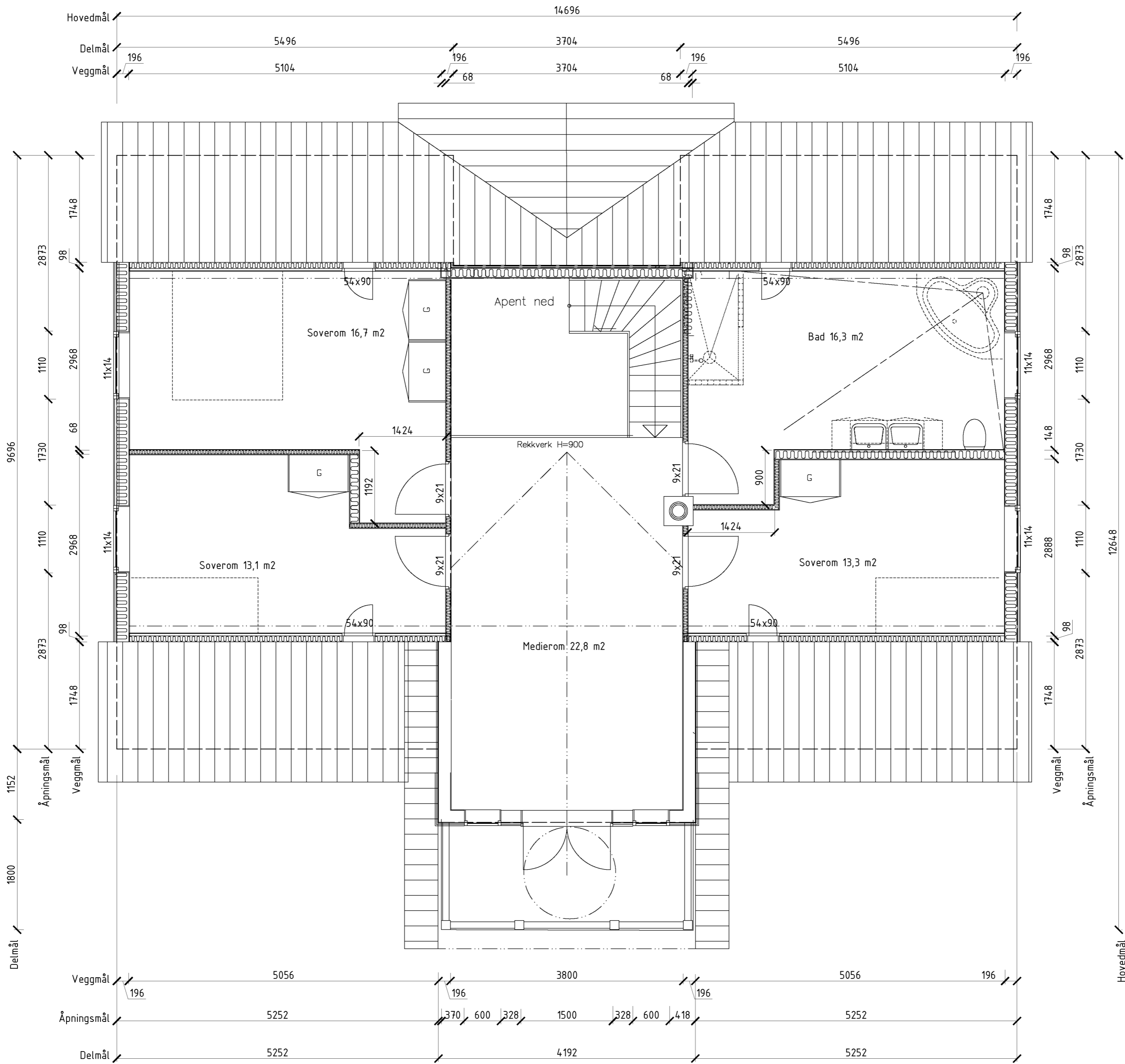
LOFTSETASJEPLAN (Oppgitt romareal = gulvflate)
