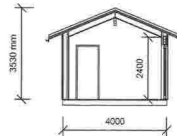
Snitt A
