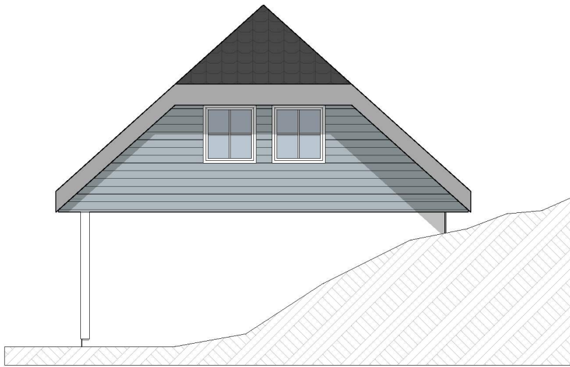
1:100 Fasade Sørøst
