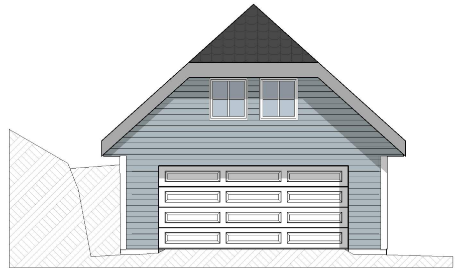
1:100 Fasade Nordvest
