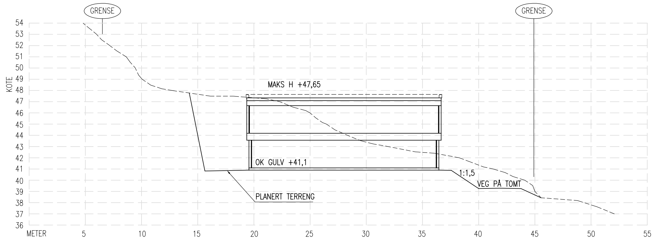
TERRENGPROFIL B-B
