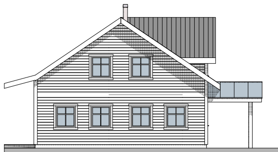
1:20 Fasade NORD-VEST
