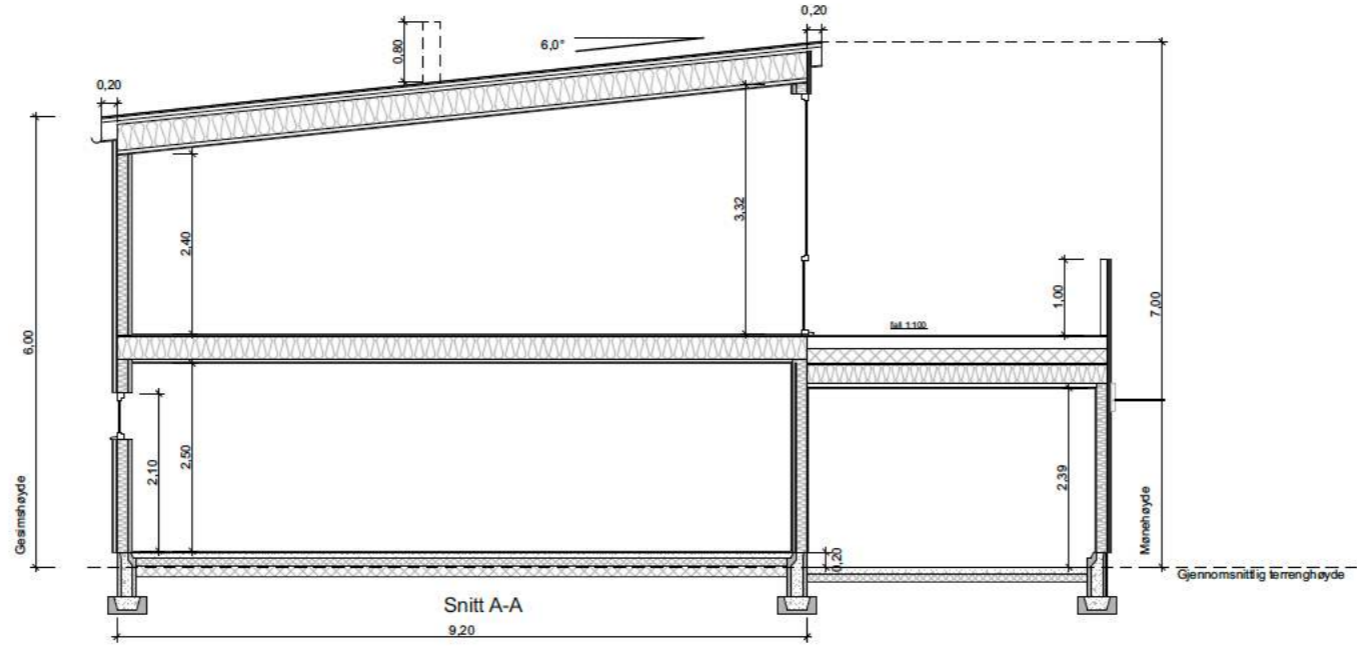
Snitt A
