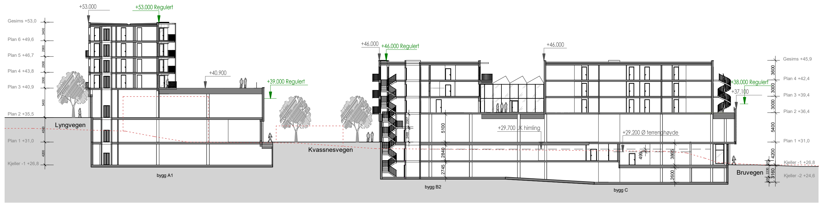
Snitt A-A (sett mot øst) 1:400
