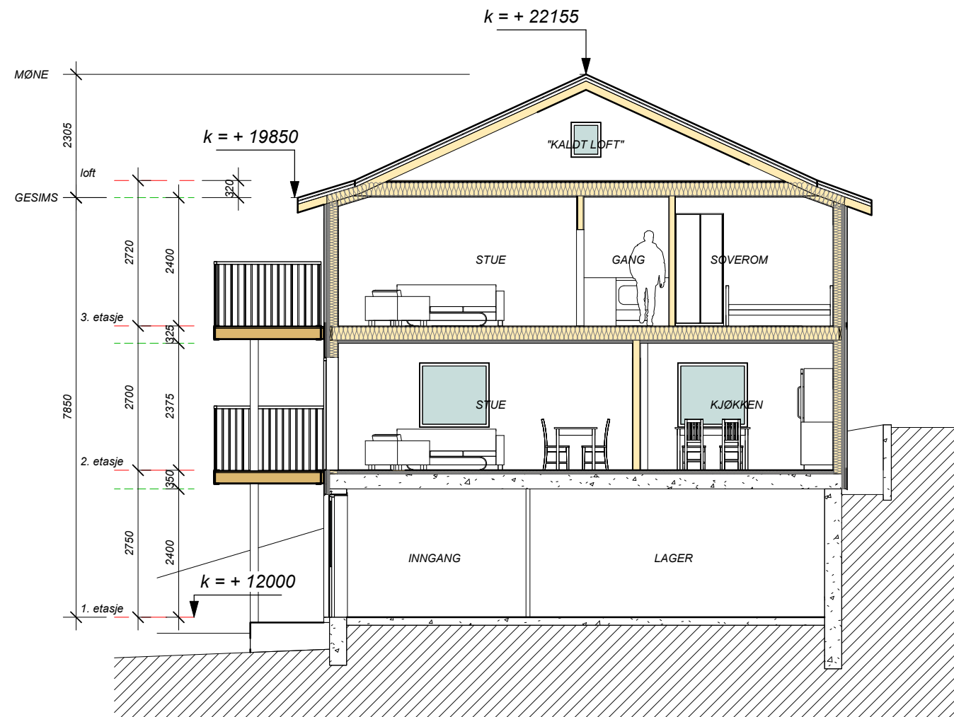
1 Snitt A-A 1 : 100
