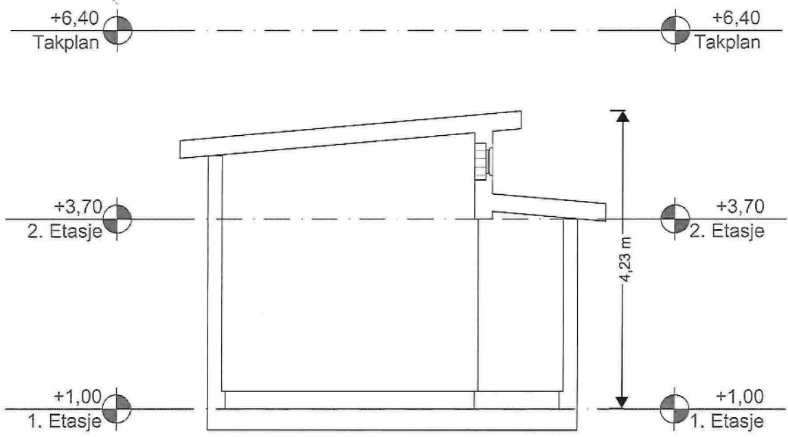
1:50 Snitt B
