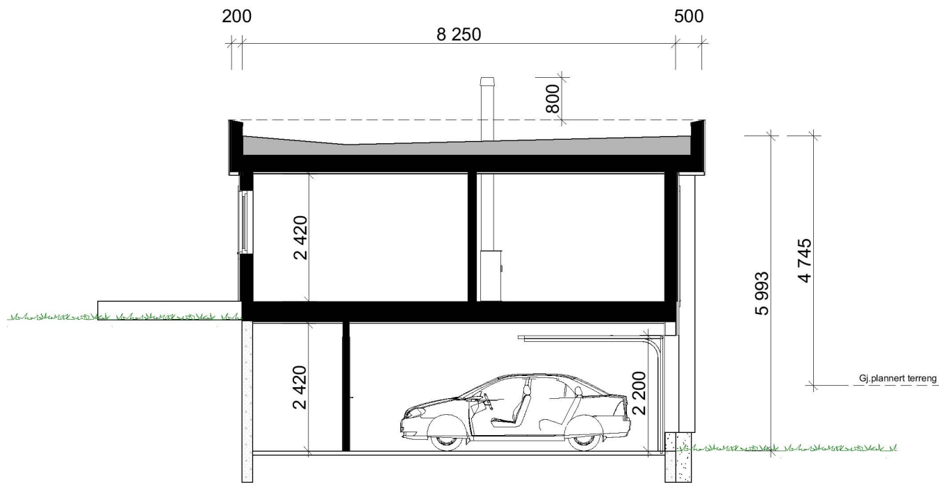
1:100 Snitt A
