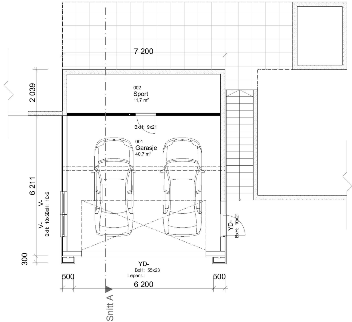
1:100 U. etasje
