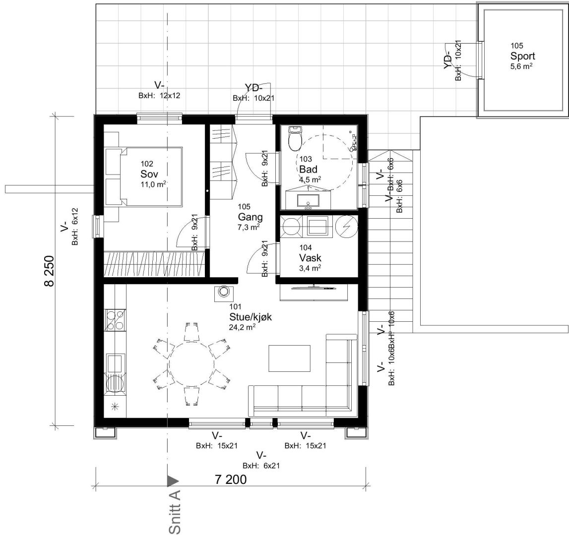
1:100 H. etasje
