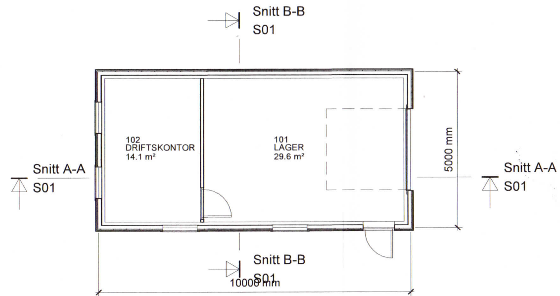
Plantegning
