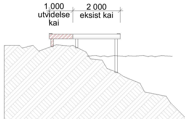
1:100 Snitt A
