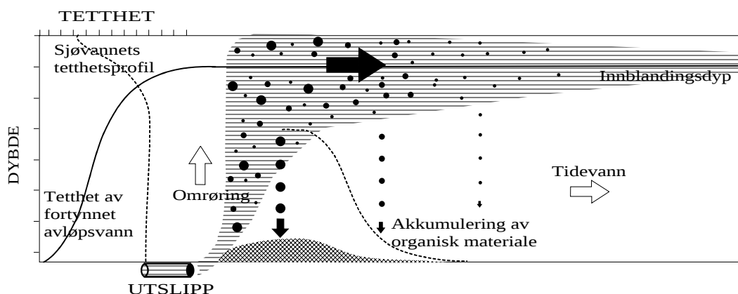
Figur 8. Prinsippkisse for primærfortynningsfasen av innblanding av et ferskvannsutslipp i en sjøresipient. Utslippet får økt sin tetthet ettersom det lettere ferskvannet stiger opp og blandes med sjøvannet (heltrukken linje).
