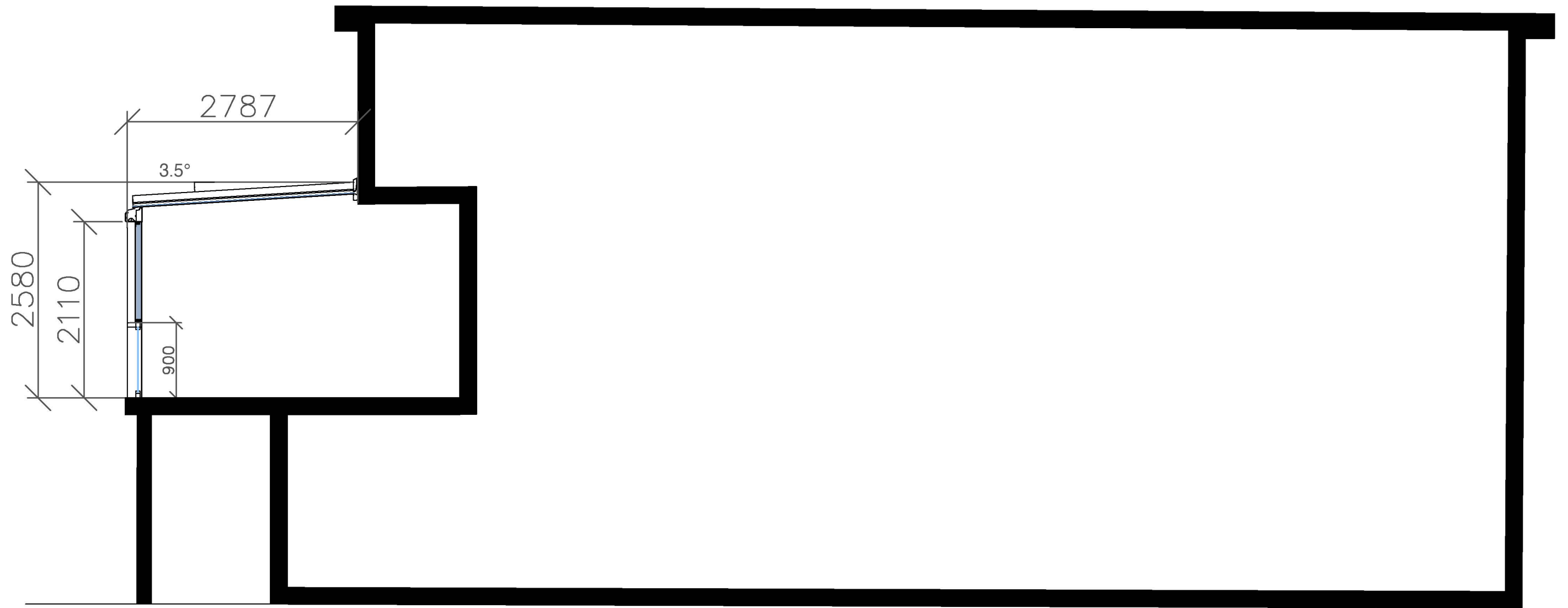
Snitt A - Utestue
