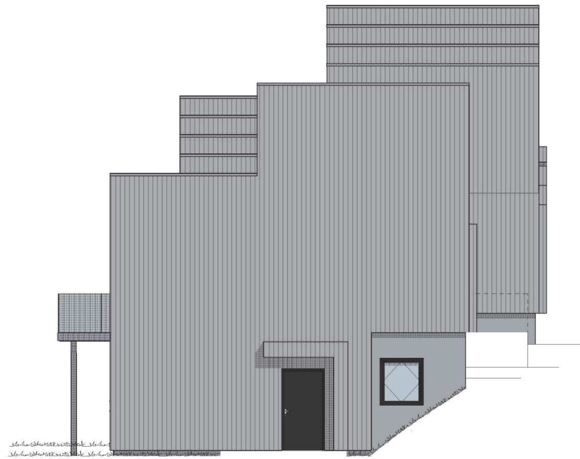
Fasade Øst
