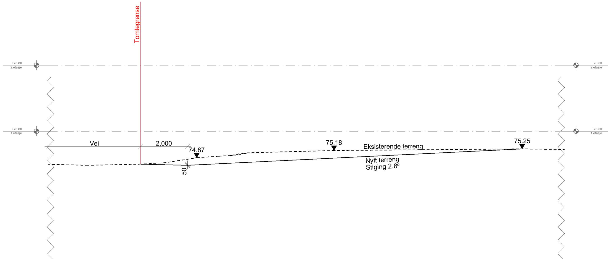
Lengdeprofil 1:100
