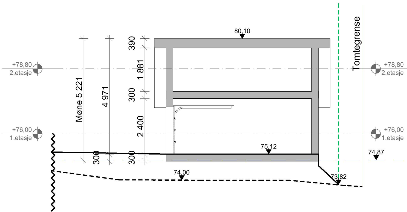
1:100 Snitt G (Garasje)
