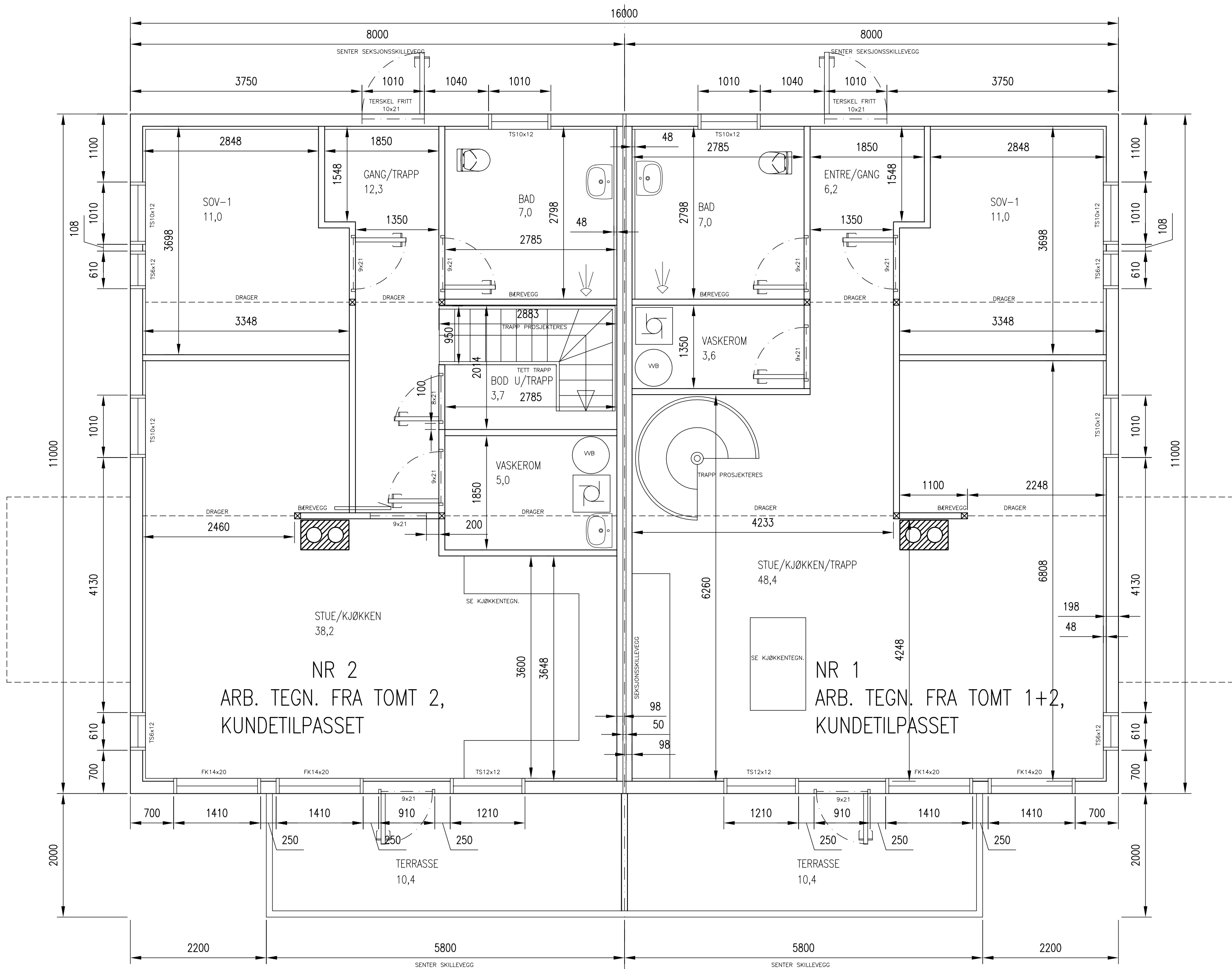
ARBEIDSTEGNING 1. PLAN
