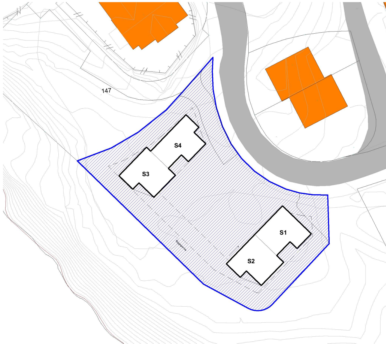
1:500 Situasjonsplan
