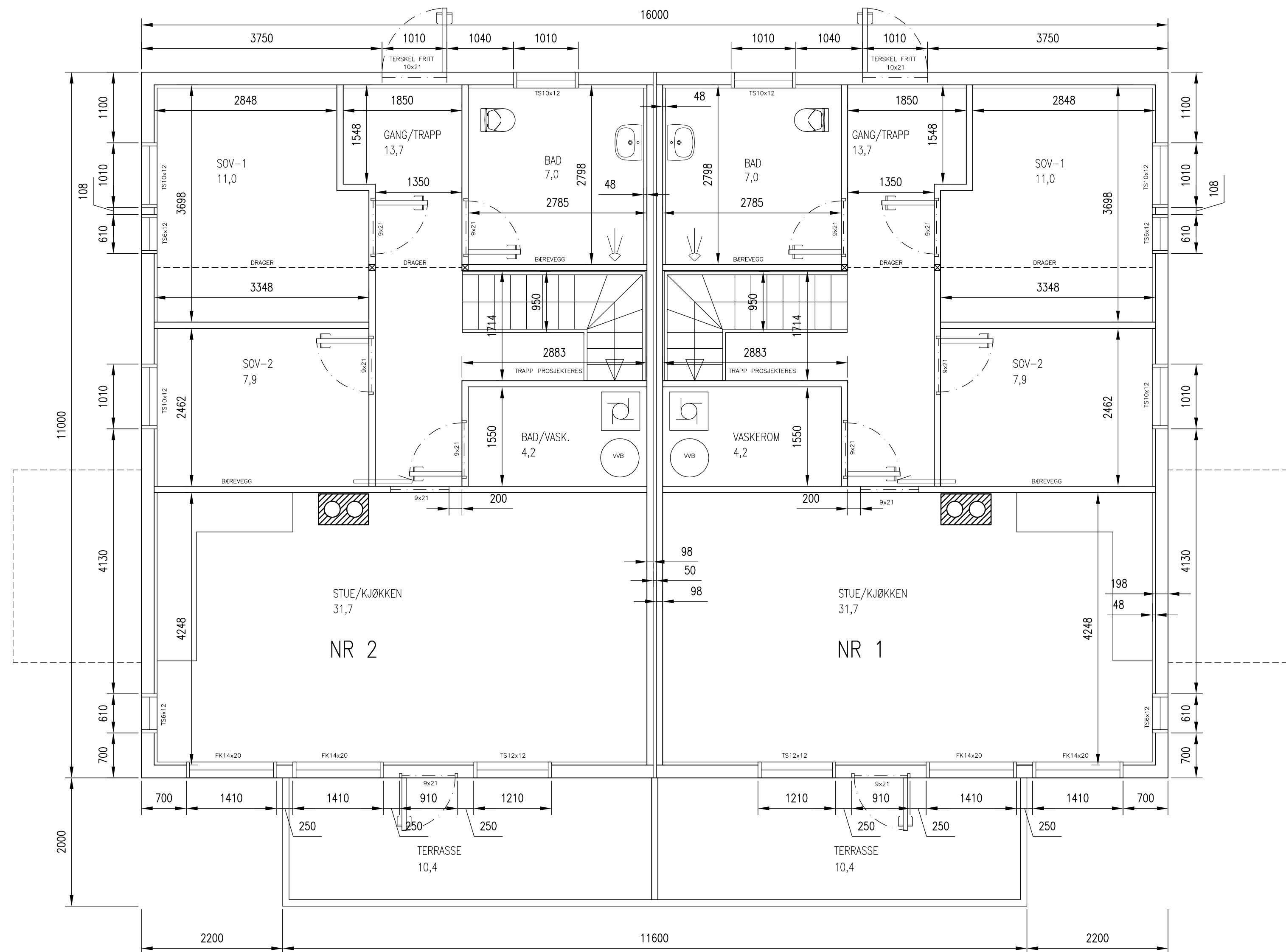
ARBEIDSTEGNING 1. PLAN
