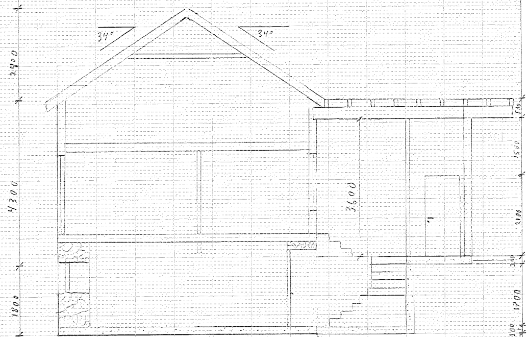
Snitt A-A
