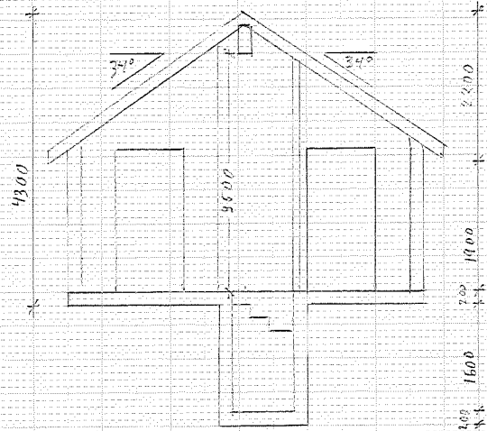
Snitt B-B
