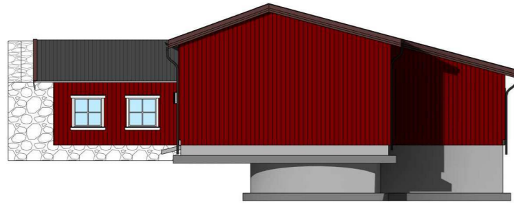
Fasade 1 1 : 100
