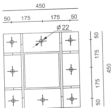
Anchors glued Hilti HY 200-A
