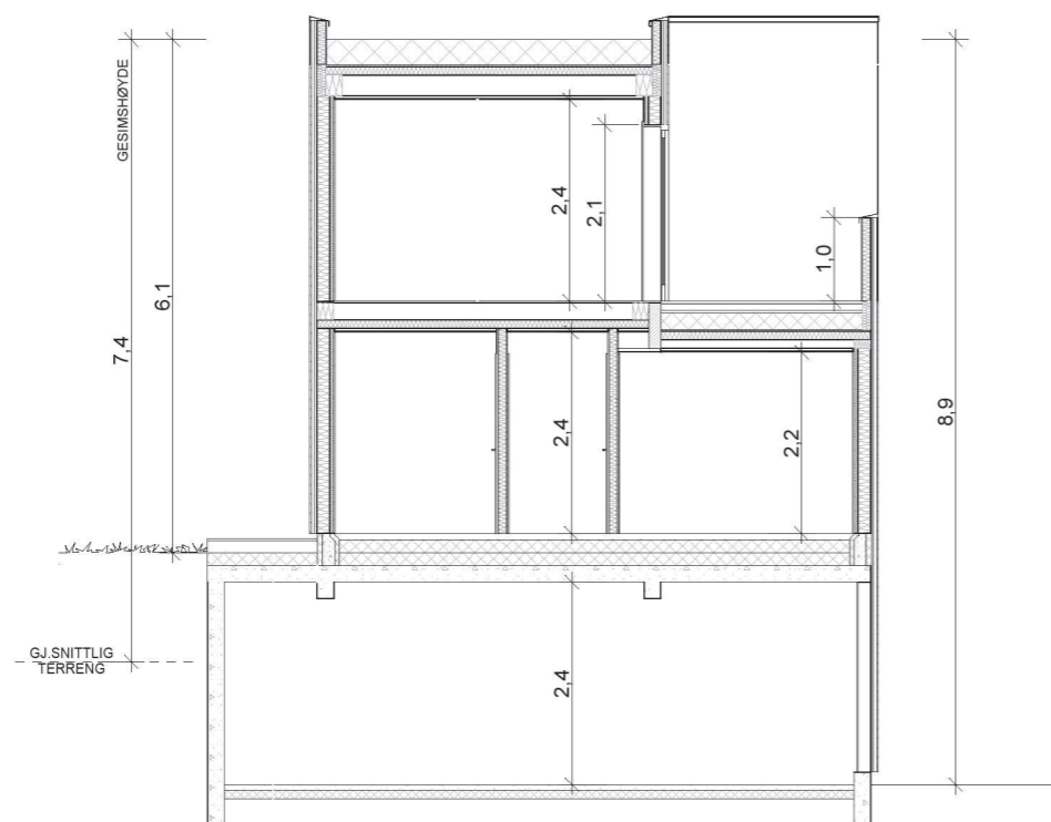
SNITT A
