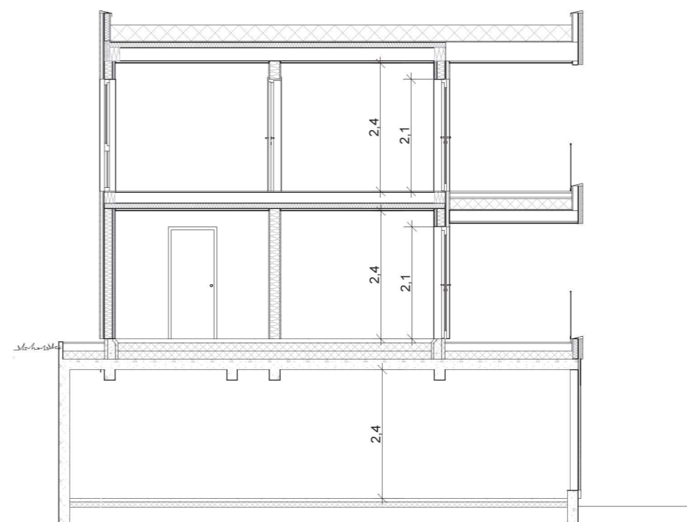
SNITT B
