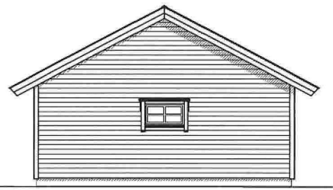
Fasade 2
