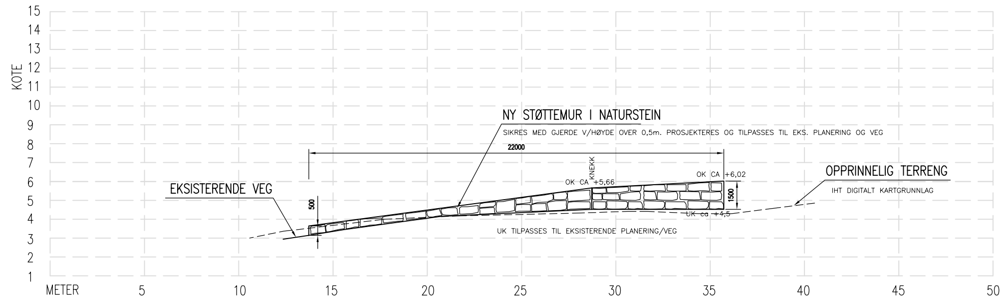
MURPROFIL 1
