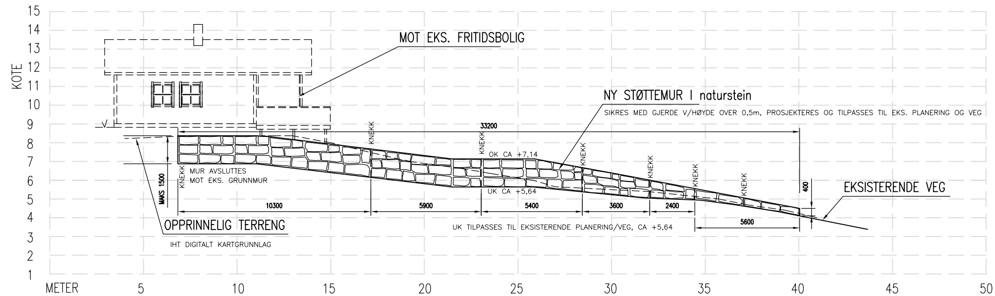
MURPROFIL 2
