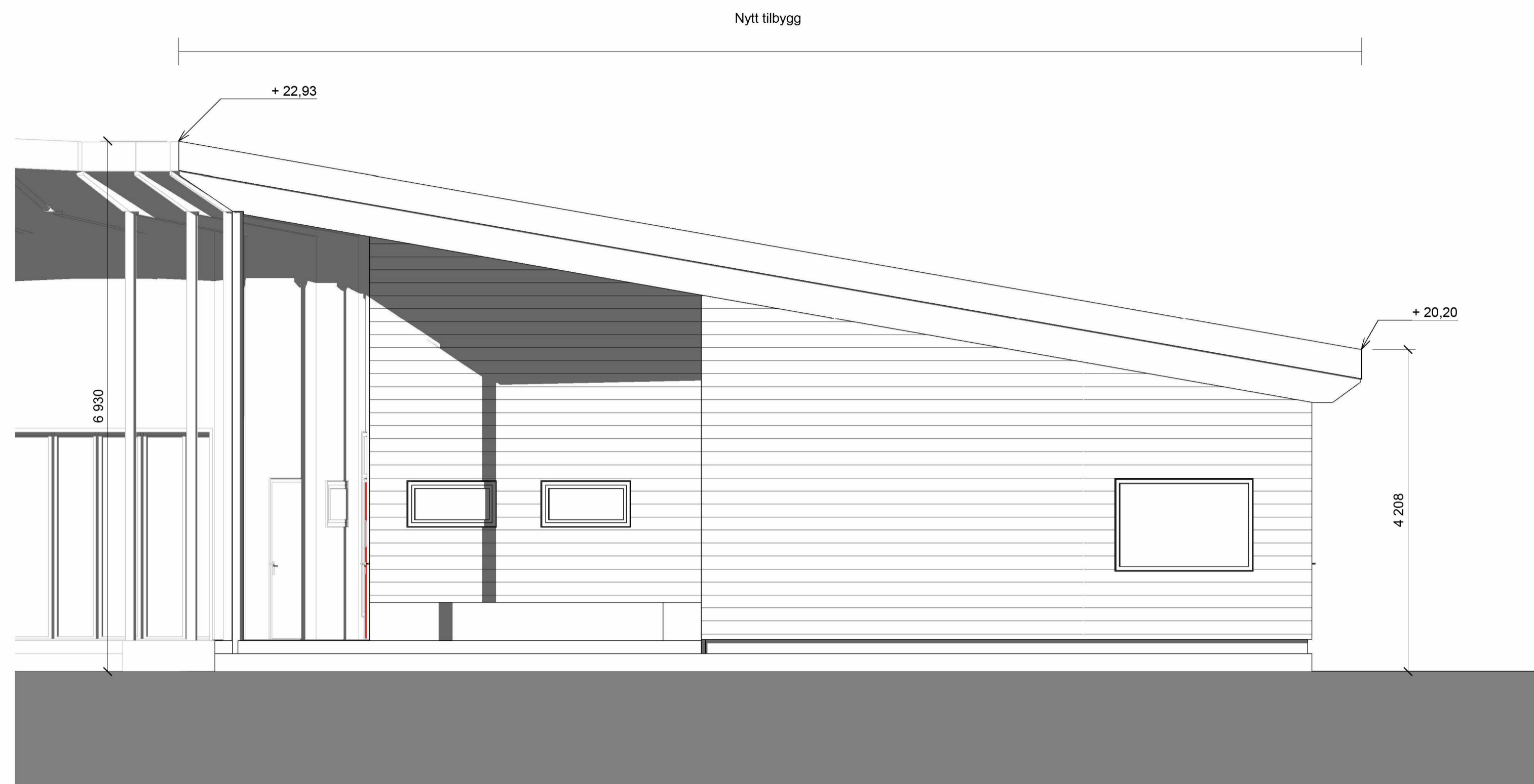
Fasade sør 1 : 50
