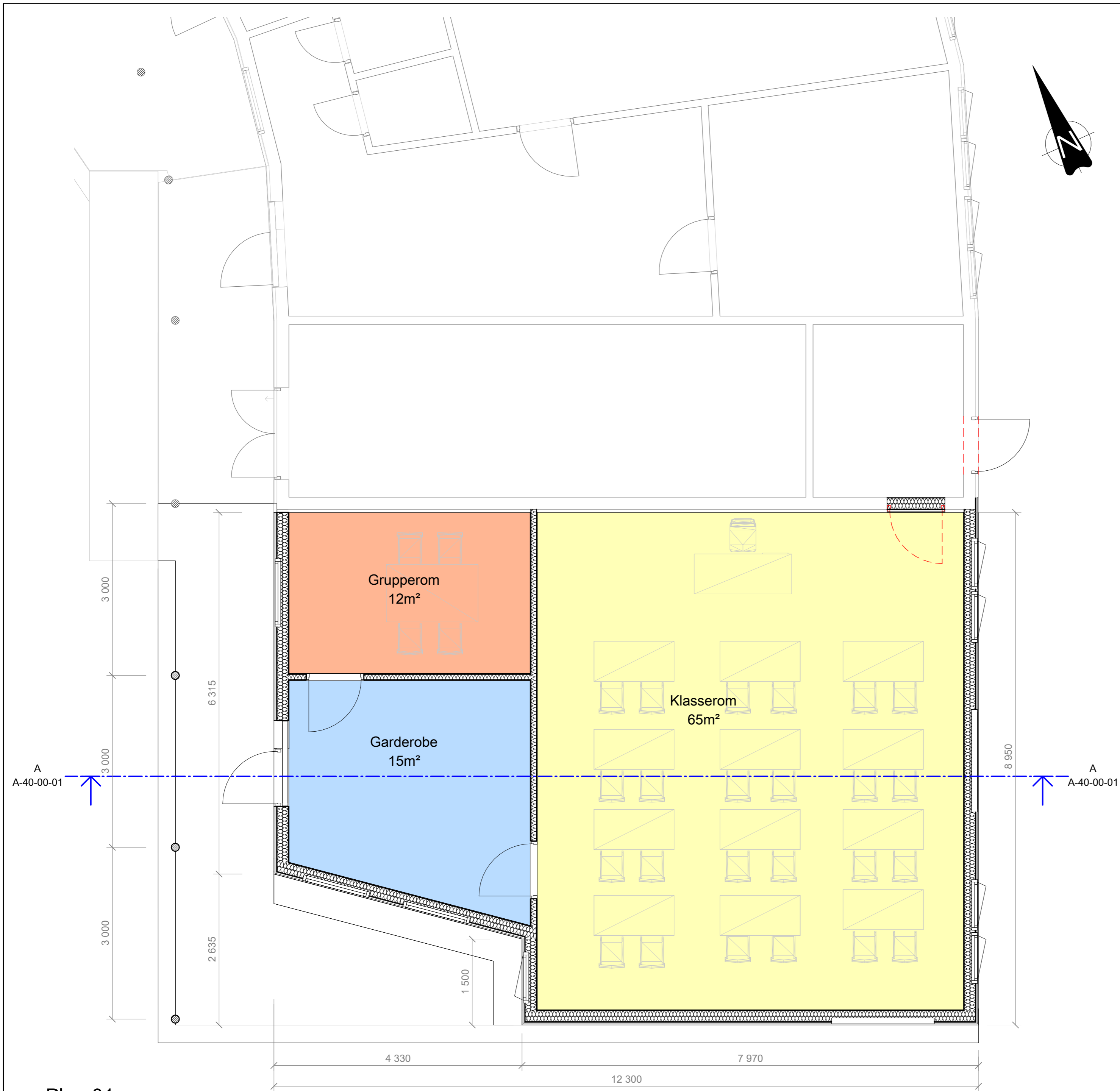
Plan 01 1 : 50
