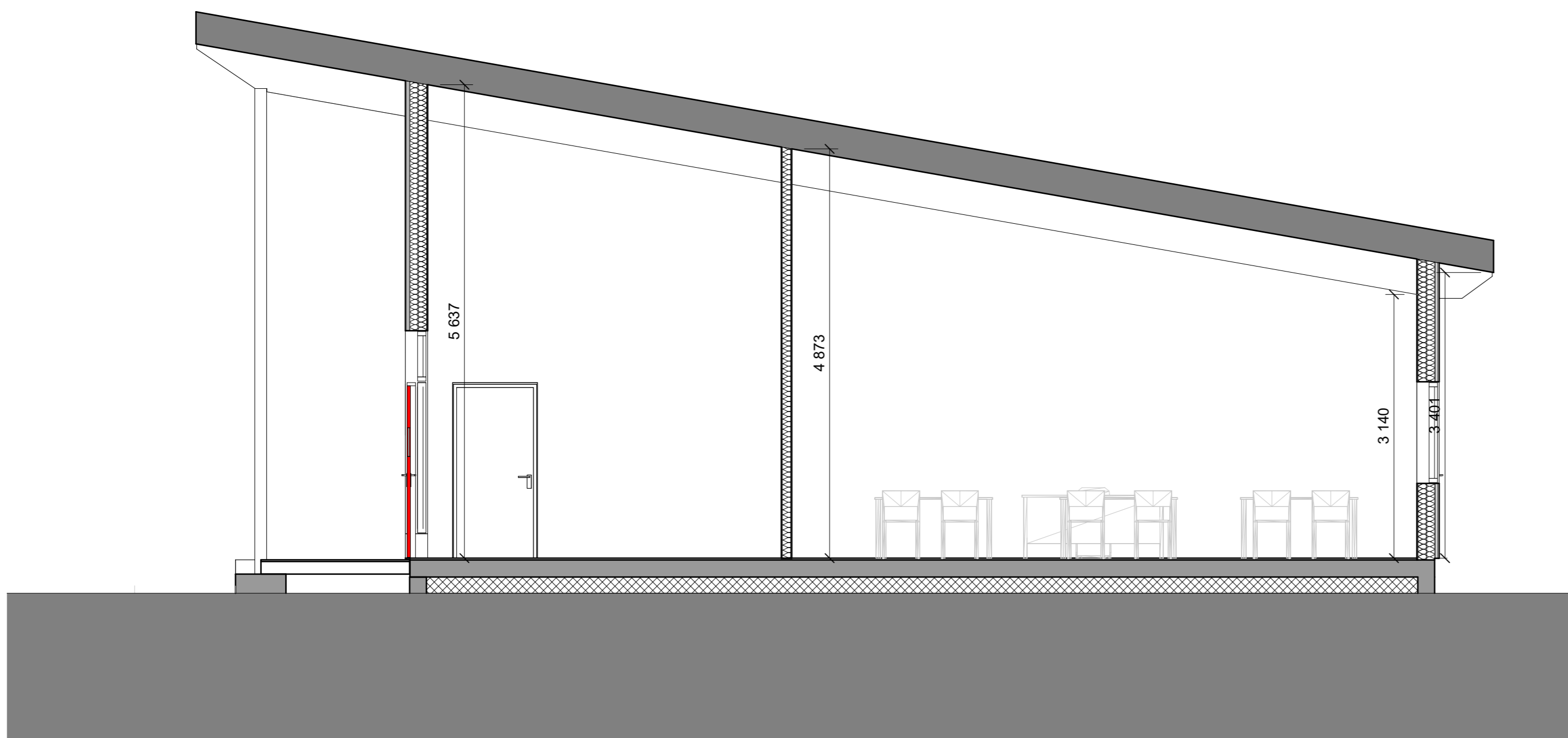
Snitt A-A
