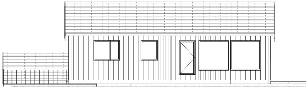
3 Vest 1 : 100
